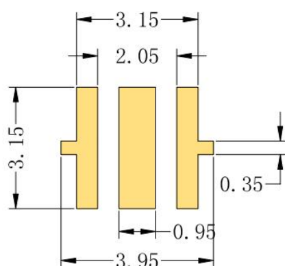
建议钢网
