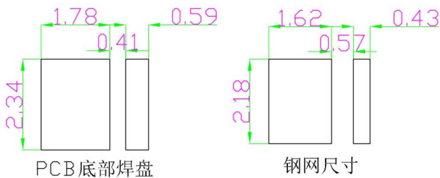
建议焊盘图
